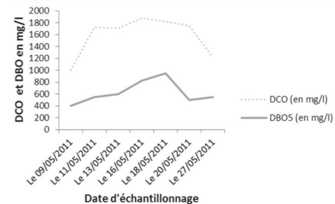
Figure 10 : Evolution de la DBO5 et de la DCO au cours du processus de compostage
